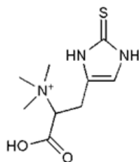
Ergothioneine
