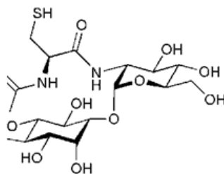
Mycothiol
